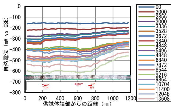
図－7 外部照合電極による自然電位の経時変化
