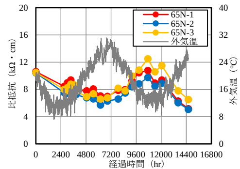
図－9 比抵抗の経時変化（65N）
