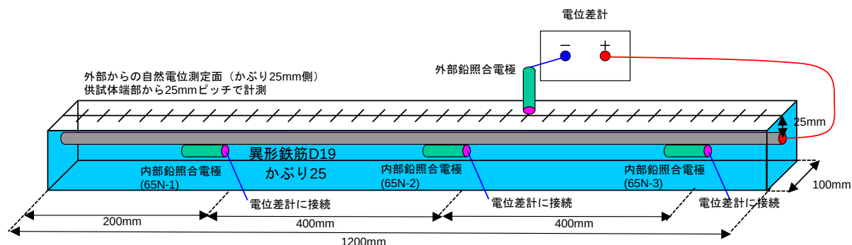
図－1 供試体の形状と自然電位の計測位置
