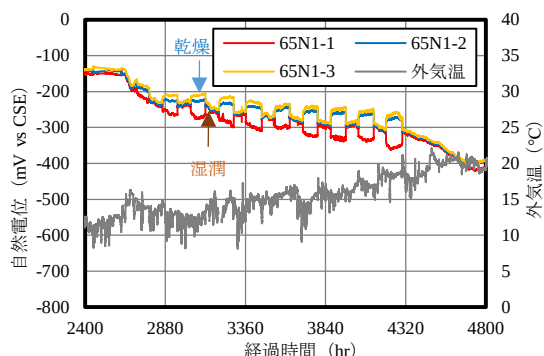
図－5 内部照合電極による自然電位の 2400-4800hr 経時変化
