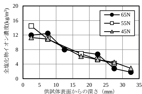
図－11 塩化物イオン濃度分布
