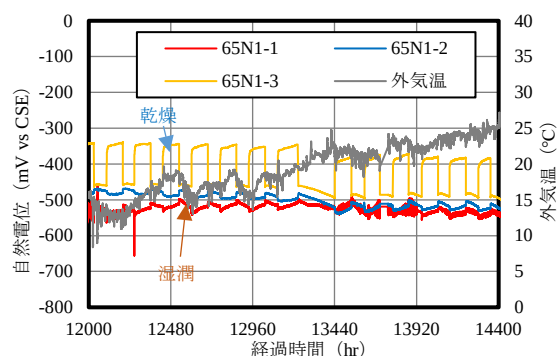
図－6 内部照合電極による自然電位の 12000-14400hr 経時変化
