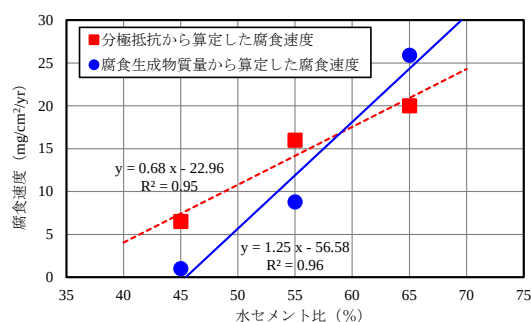
図-12 水セメント比と腐食速度の関係
