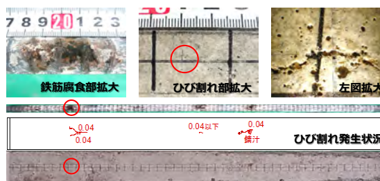
図－10 鉄筋腐食および腐食ひび割れの発生状況
