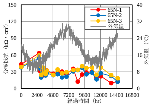
図－8 分極抵抗の経時変化（65N）
