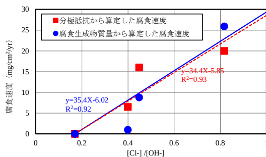
図-13 [Cl^-]/[OH^-] と腐食速度の関係
