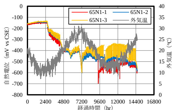
図－4 内部照合電極による自然電位の 0-14592hr 経時変化
