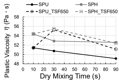
図-8 空練り時間と塑性粘度の関係
