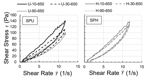
図-5 ヒステリシスループ（同一目標スランプフロー）
