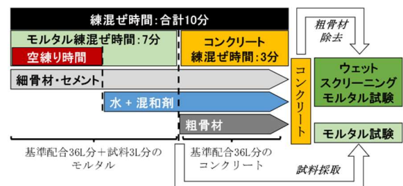
図-1 練混ぜ方法
