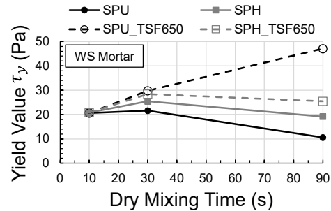
図-14 空練り時間と降伏値の関係
