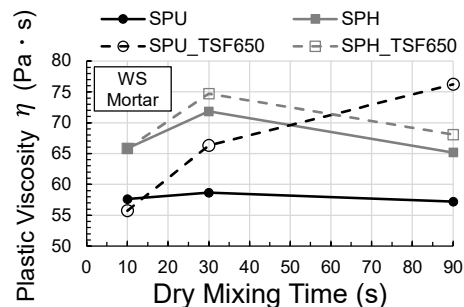
図-15 空練り時間と塑性粘度の関係
