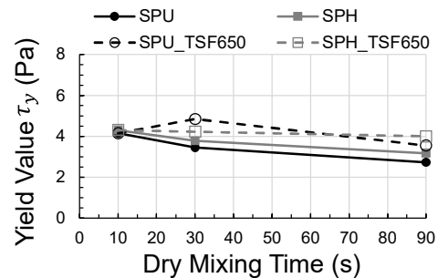
図-7 空練り時間と降伏値の関係
