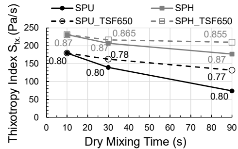
図-6 空練り時間とチクソトロピー指数 s_{tx} の関係
