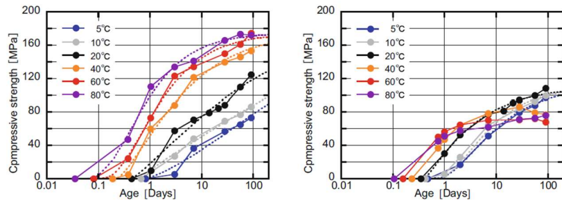
図一六 既報 12) の結果 (左 : STC-Zero, 右 : H-Con)
