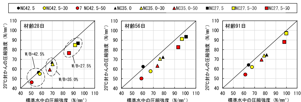
図-4 標準水中養生強度と 20°C封かん養生強度の関係
