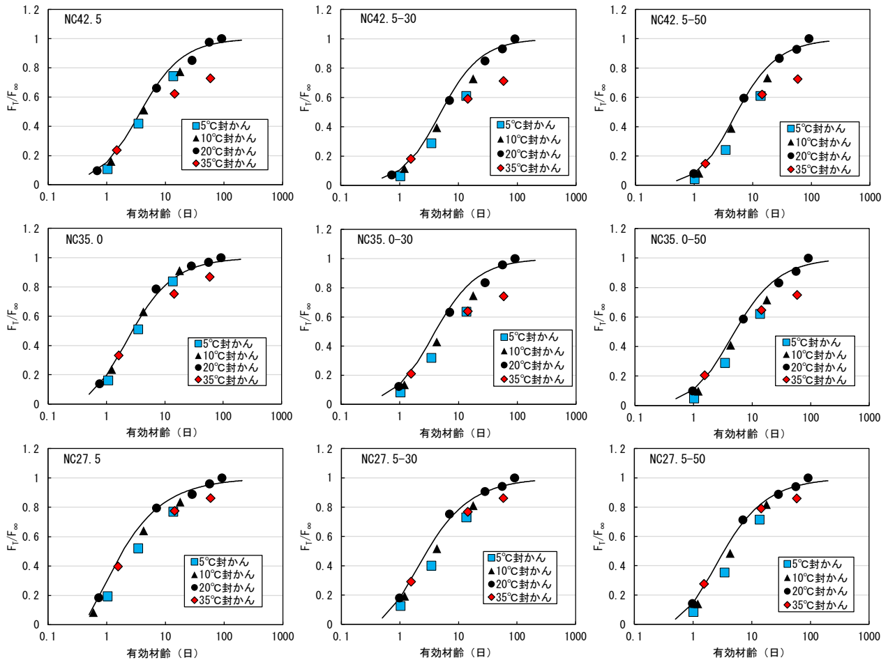
図一五 有効材齢 ( E_a=33.5\text{kJ/mol} ) と F_\infty に対する比率の関係 (5, 10, 20, 35°C 封かん)
