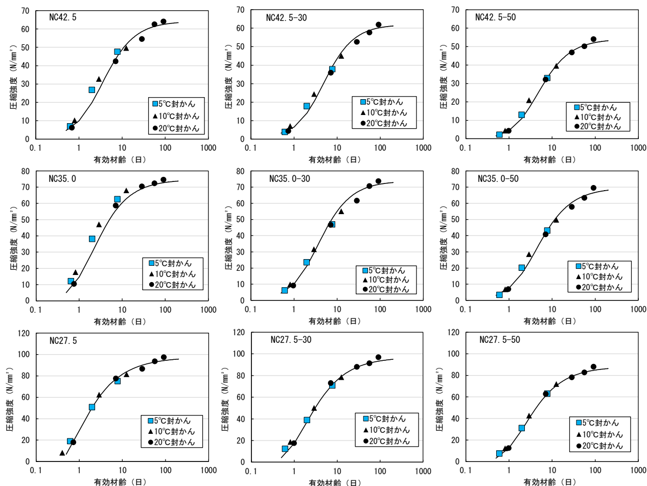
図-7 有効材齢 ( E_a=60\text{kJ/mol} ) と圧縮強度の関係 (5, 10, 20°C封かん)
