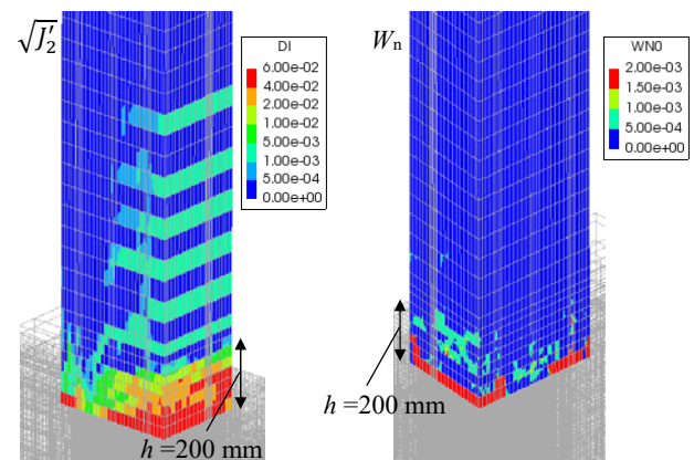
図－13 コンクリートの損傷結果（ 8\delta_y ）
