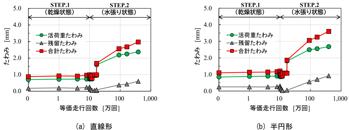
図-4 等価走行回数 N_{eq} と床版中央のたわみ
