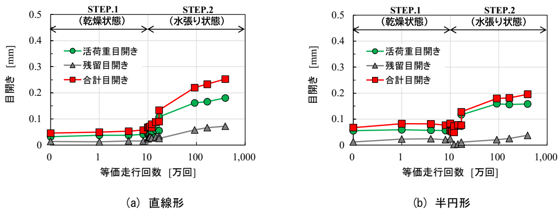
図-5 等価走行回数 N_{eq} と目開き
