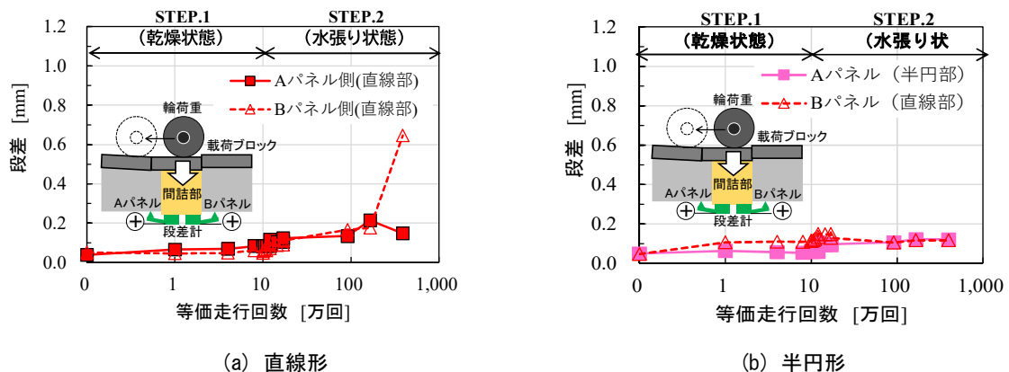
図-6 等価走行回数 N_{eq} と段差
