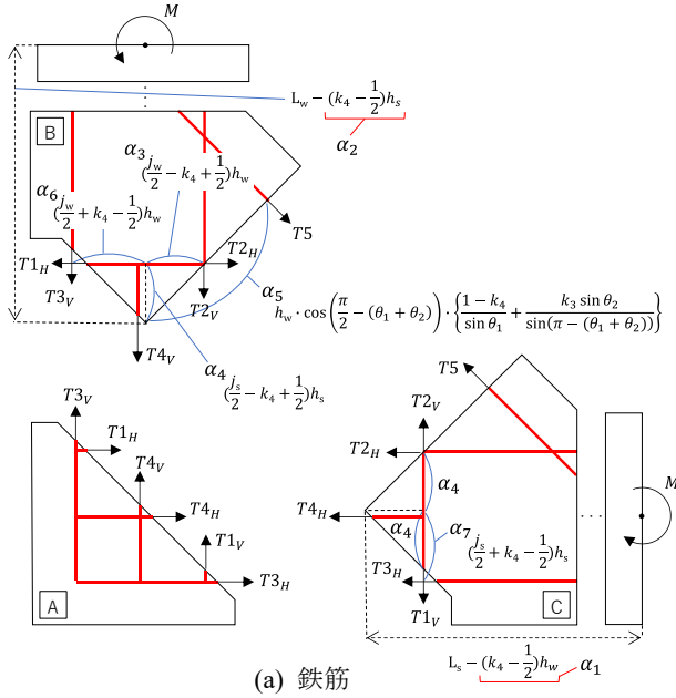
図-9 分割モデルにおいて作用する力の定義
