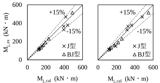
図-11 実験値と計算値の比較
