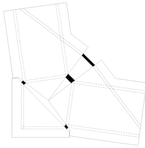
図-7 正曲げを受ける隅角部の分割モデル
