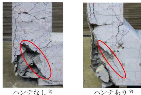
写真-1 割裂ひび割れの発生位置
