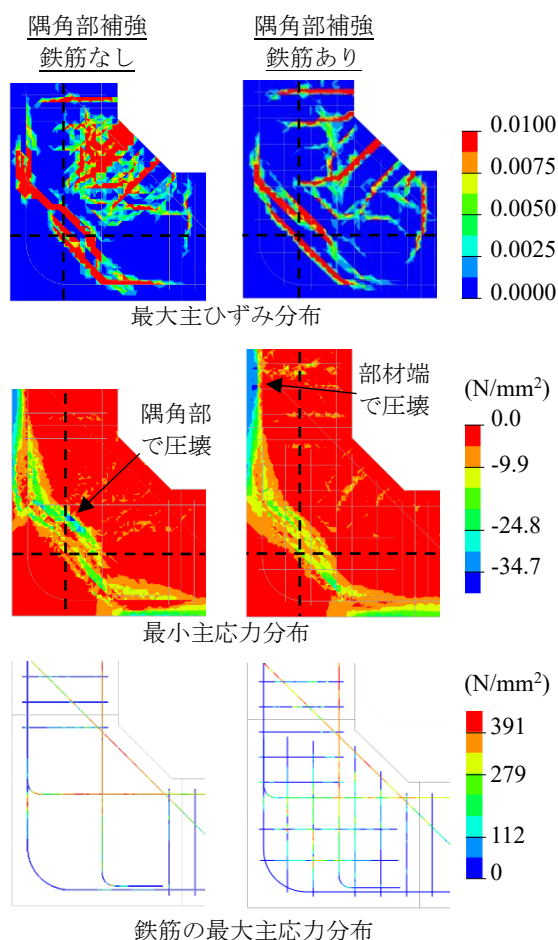
図-6 最大荷重時の応力・ひずみ分布
