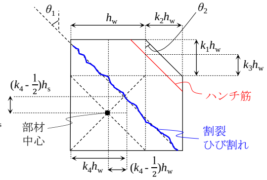
図-8 記号の定義
