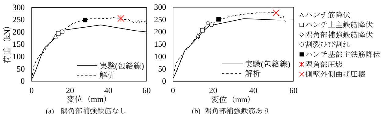
図-5 解析結果（荷重－変位関係）
