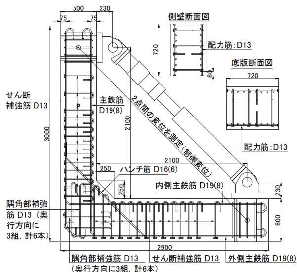
図-1 試験体諸元 (Case1)
