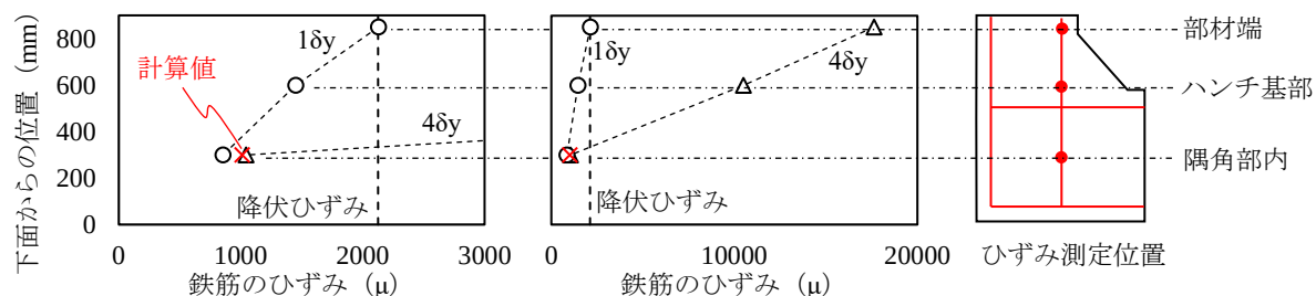
図-4 側壁内側主鉄筋のひずみ分布
