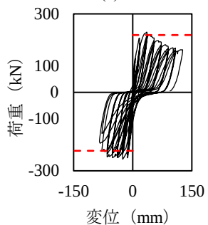
(b) 隅角部補強鉄筋なし (Case4)
