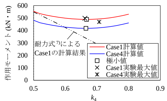
図-10 作用モーメントに与える k_4 の影響
