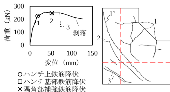
図-3 包絡線およびひび割れ性状 (Case1)
