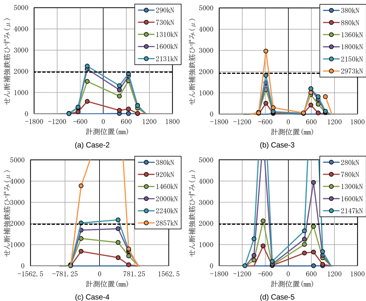
図-4 せん断補強鉄筋のひずみ分布
