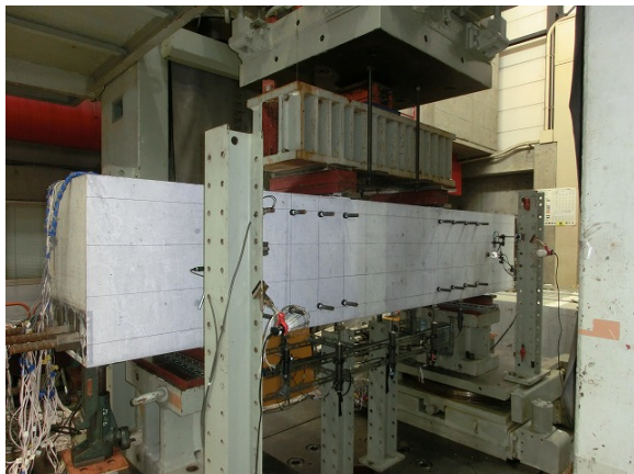
写真-2 荷重試験状況
