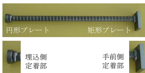
写真-1 後施工プレート定着型せん断補強鉄筋
