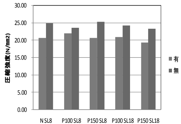
図－６ 反発度法による圧縮強度結果
