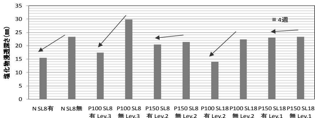
図－５ 塩化物浸透深さ結果
