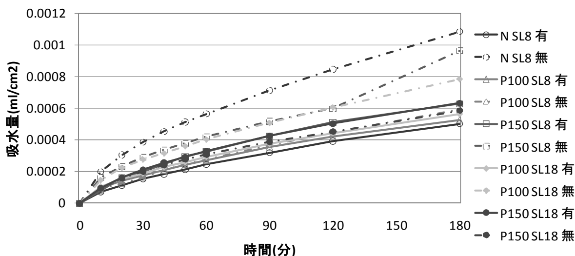
図－2 吸水量試験結果
