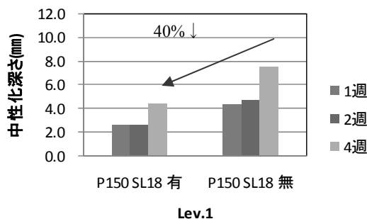
図－4 促進中性化試験
