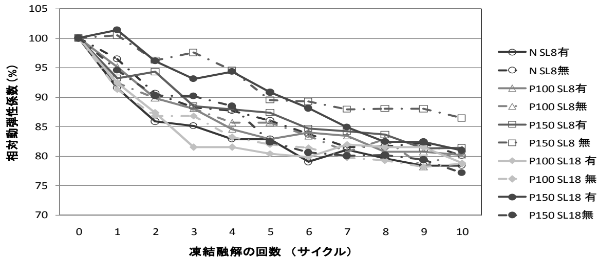
図ー 7 急速凍結融解試験結果
