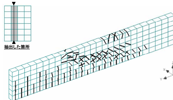
(b)構造物内部のひび割れ状況
