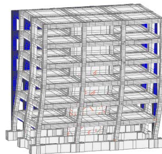
図-16 6階建てRC造建築の非線形動的解析
