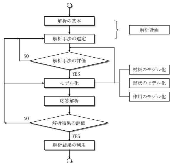
図－1 非線形有限要素解析の評価と利用のフロー
