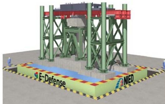
図－12 実物大橋脚振動実験
