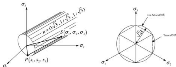
図-4 von Mises モデル 3.3.2 鋼
