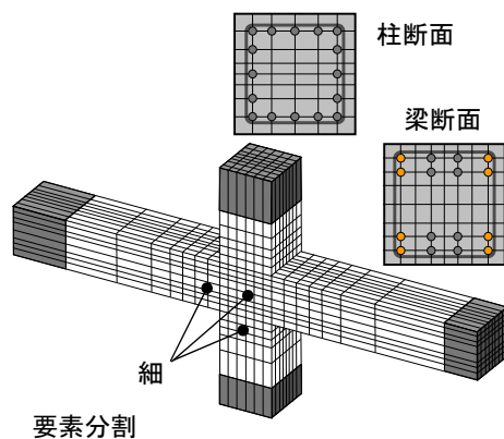
図－10 トライ＆エラーにより導かれた標準的なモデル
