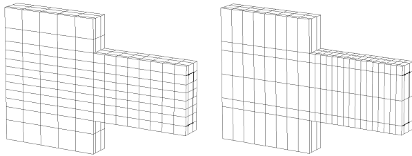
(a) 適切な分割 (b) 不適切な分割
