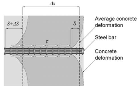
図-6 鉄筋とコンクリート間の付着滑り
