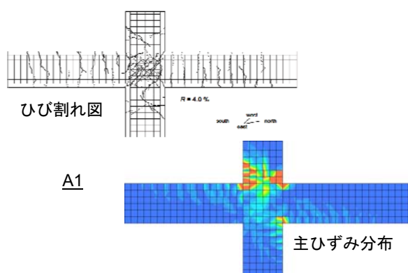
(b) 損傷状況の比較
