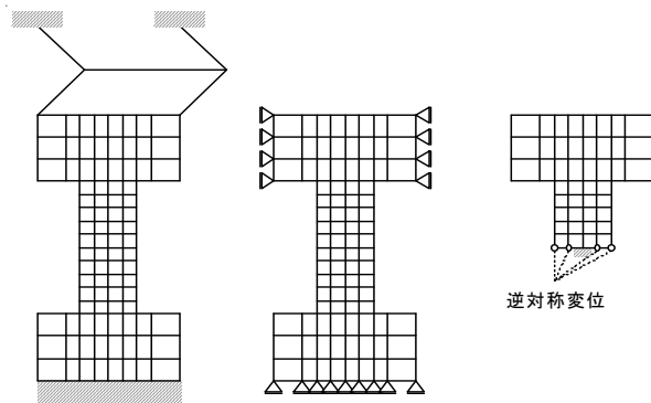
図-3 柱試験体の境界条件
