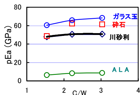
図-2 見掛けの弾性係数(pEa)と(C/W)
