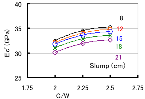
図-6 コンクリートの弾性係数 ( E_c' ) とセメント水比
