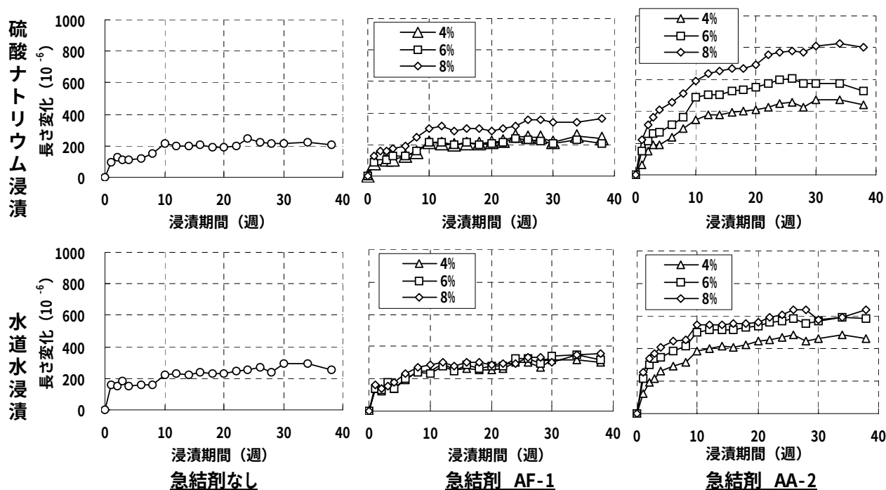
図-3 浸漬期間と長さ変化の関係（浸漬開始材齢 1 日）
