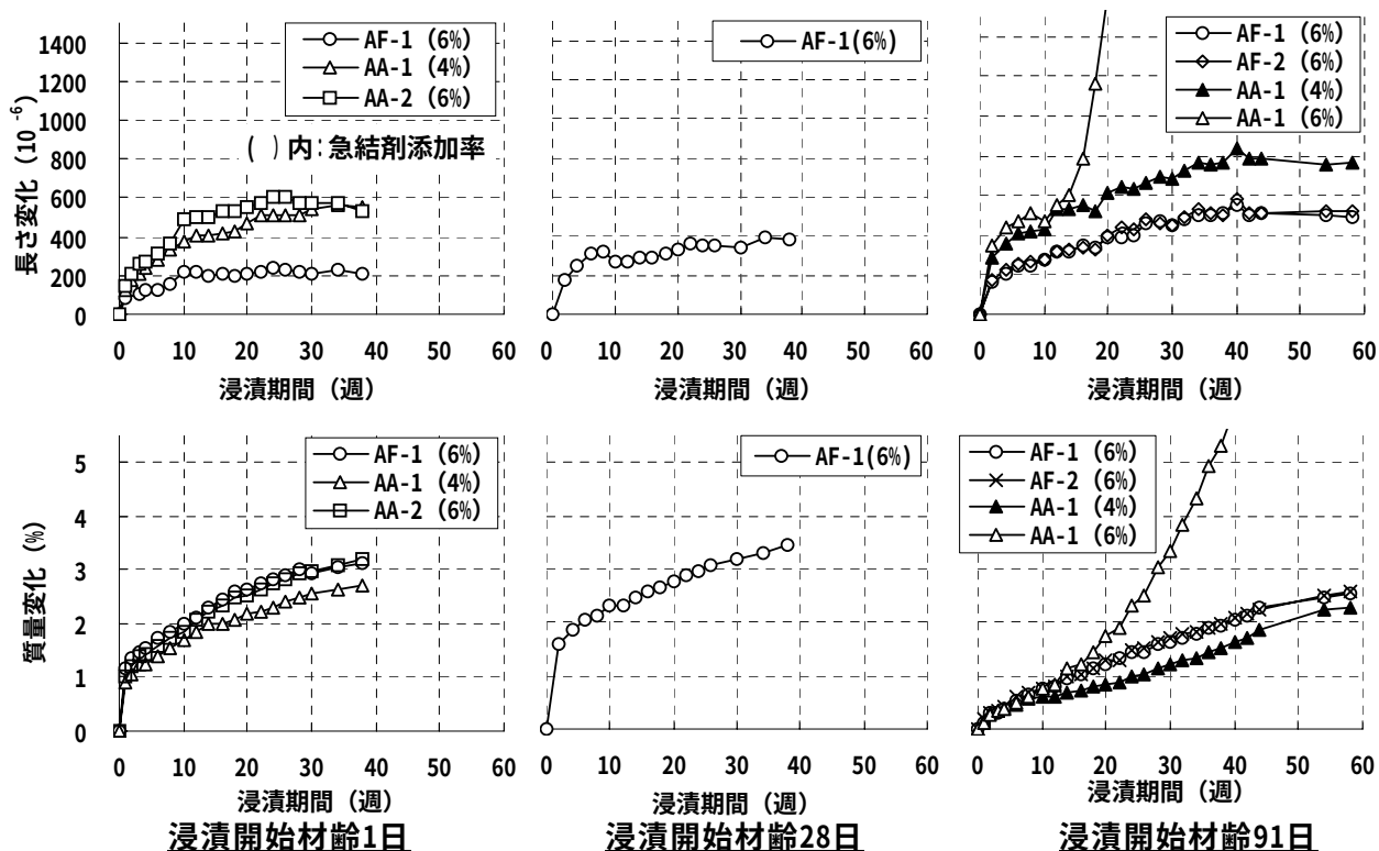
図-2 浸漬期間と長さ変化・質量変化の関係（硫酸ナトリウム 10%溶液浸漬）
