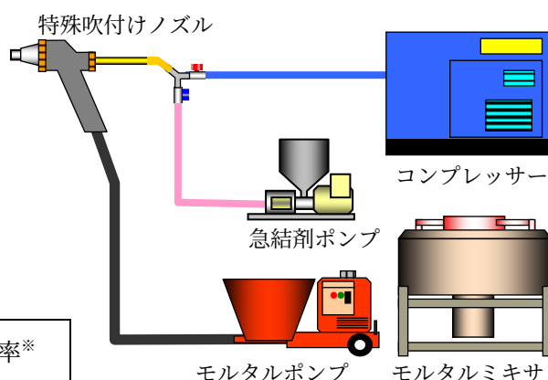
図－１ 吹付けシステムの概要
