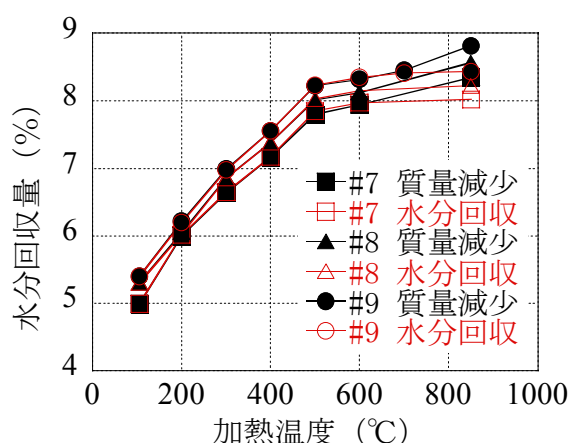
図-2 温度と化学的結合水率との関係
