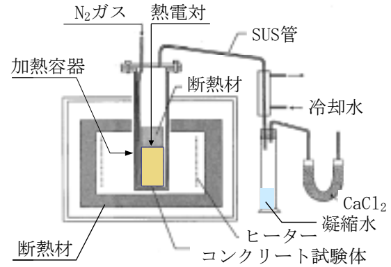
図-1 水分回収装置の概要
