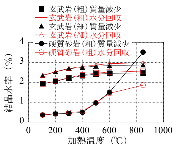
図-3 温度と結晶水率との関係
