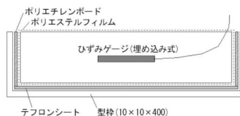
図-1 自己収縮ひずみの測定方法
