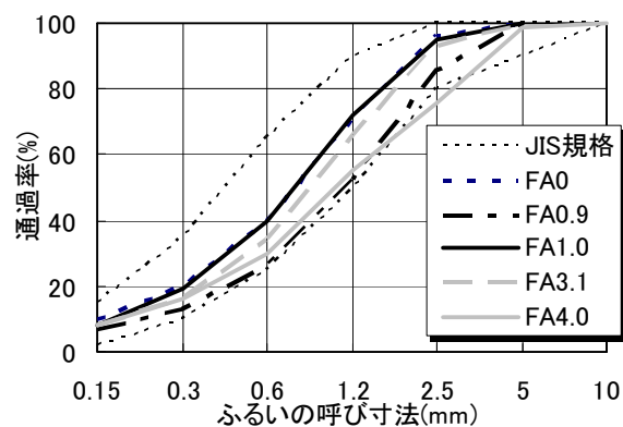
図－2 使用細骨材の粒度分布
