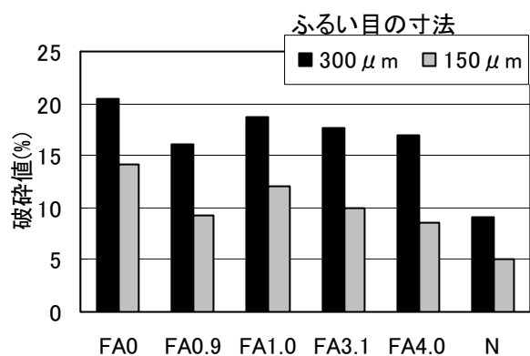
図－5 破砕値試験結果
