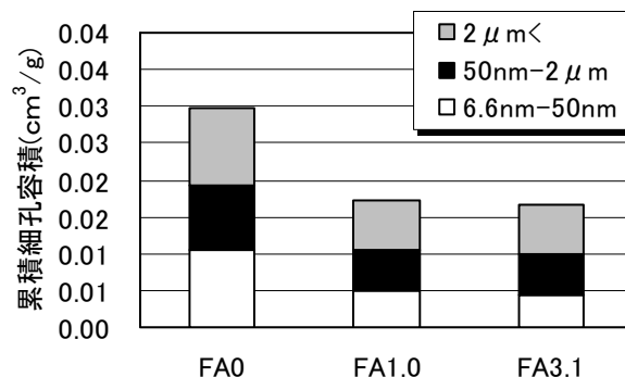
図－3 使用細骨材の細孔容積
