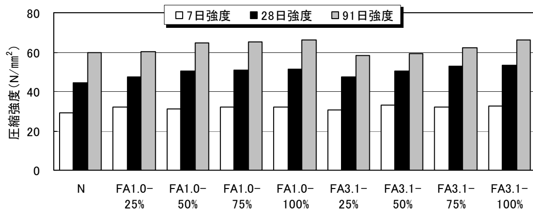
図-13 圧縮強さ試験結果
