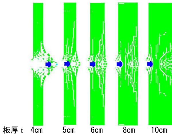
図—10 板厚による局部破壊の相違(衝突速度 300m/s)
