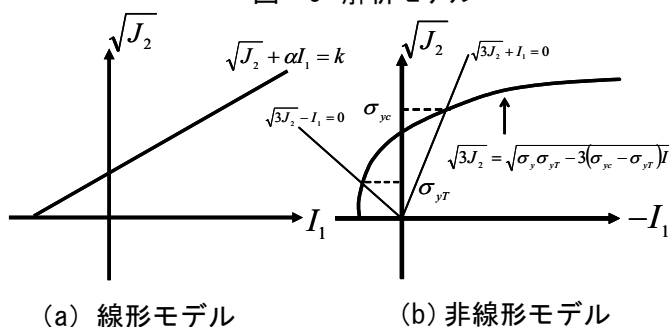
図—6 Drucker-Prager の降伏条件
