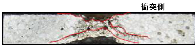
写真—3 断面の破壊状況(裏面剥離)
