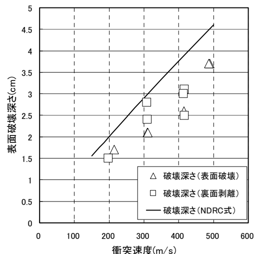
図—4 衝突速度～表面破壊深さ関係
