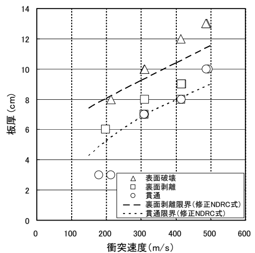
図—3 衝突速度による破壊モードの推移
