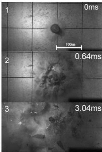
写真—4 表面破壊の映像
