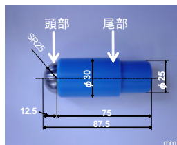
写真—1 剛飛翔体
