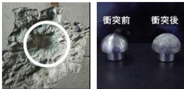
(a) コンクリート板接触部 (b) 飛翔体頭部
