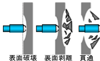
図—2 局部破壊モードの区分
