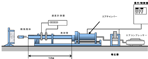
図—1 高圧空気式飛翔体発射装置
