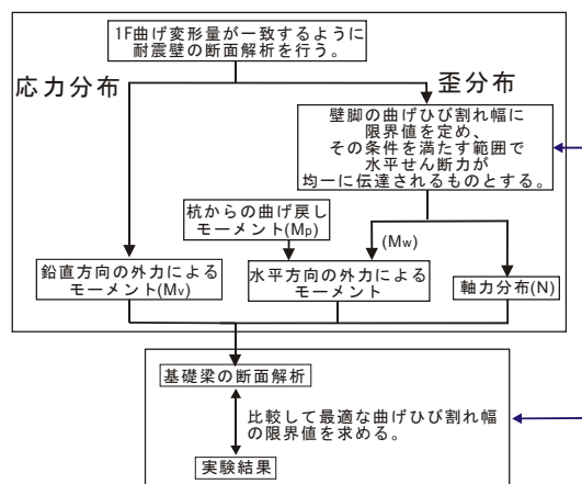
図-7 解析モデルのフローチャート
