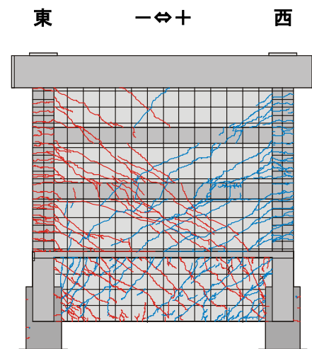
図-3 載荷終了後のひび割れ分布
