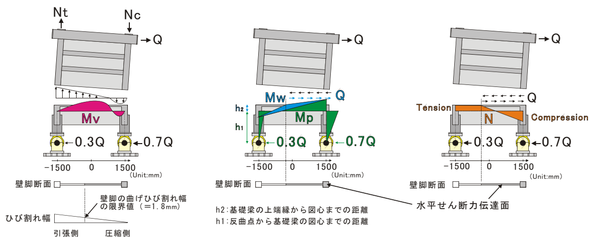
(a) 鉛直方向外力によるモーメント (b) 水平方向外力によるモーメント (c) 軸力
