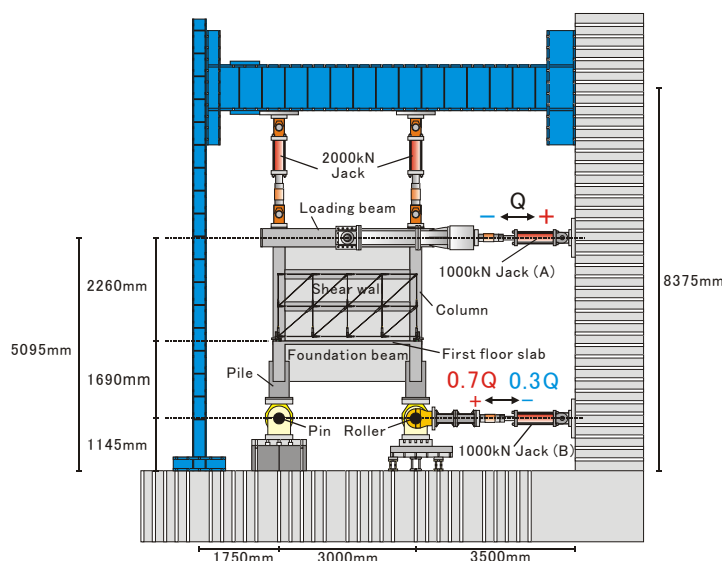
図-2 実験載荷図
