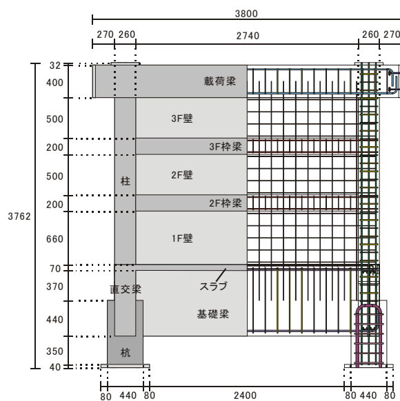
(a) 側面図及び配筋図
