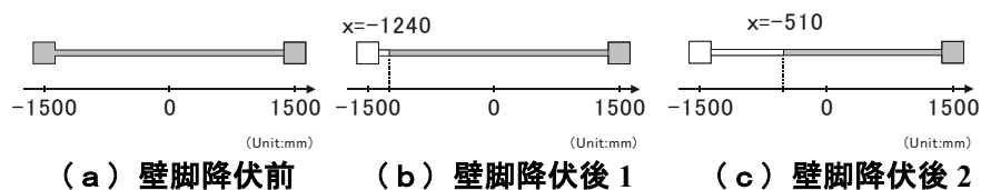
図－6 水平せん断力伝達面積の推移
