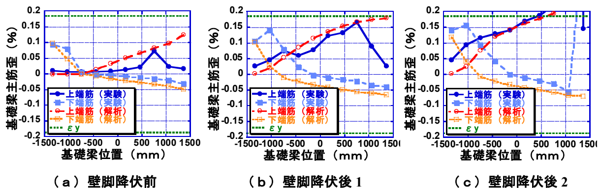
図－5 基礎梁主筋の歪分布及び断面解析の結果
