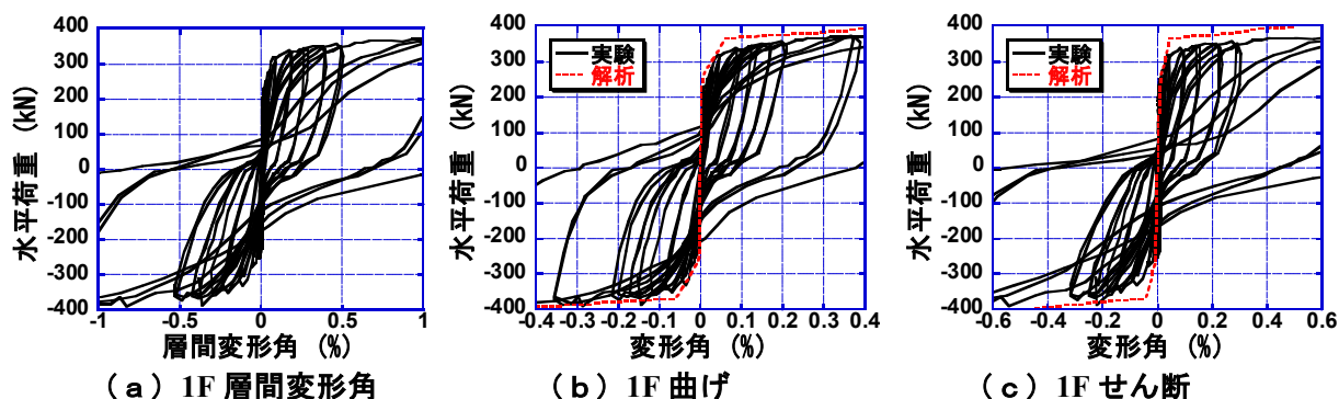
図－4 復元力特性
