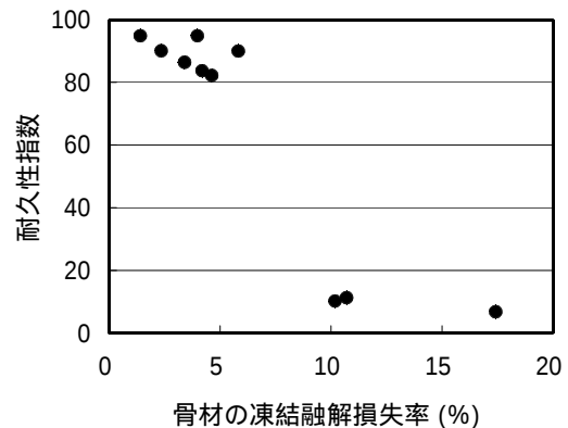
図 - 3 本試験法の結果と耐久性指数の関係 2)
