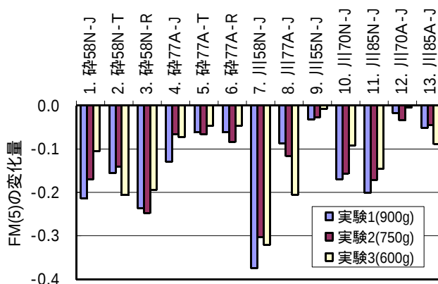
図 - 4 各再生骨材ごとのFM(5)の結果
