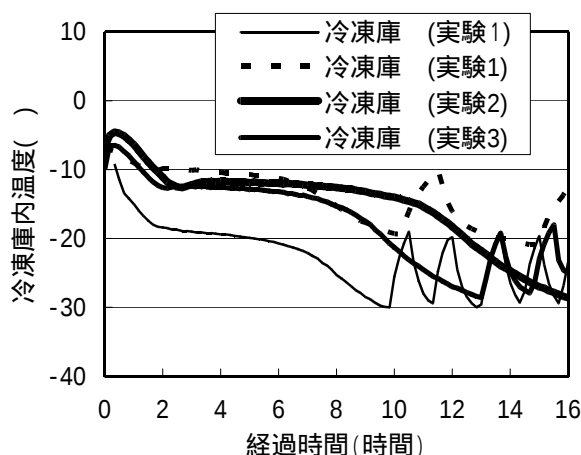
図 - 7 冷凍庫内の温度履歴
