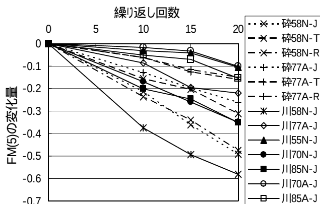
図 - 10 繰り返し回数とFM(5)の変化量の関係
