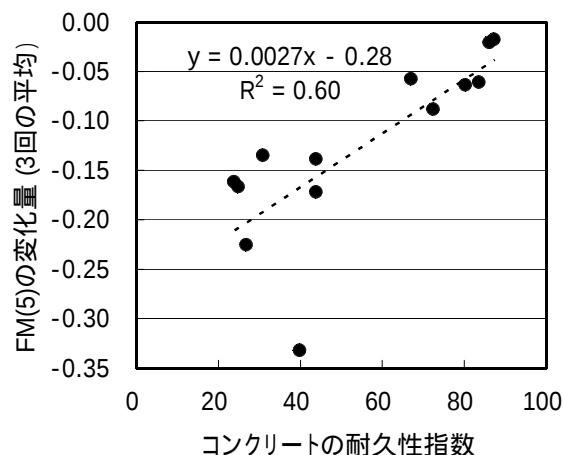
図 - 5 耐久性指数とFM(5)の関係
