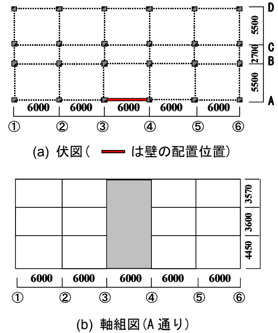
図-3 建物形状
