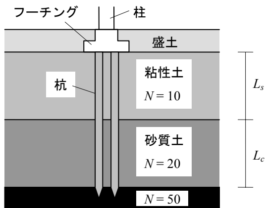
図-1 地盤構成
