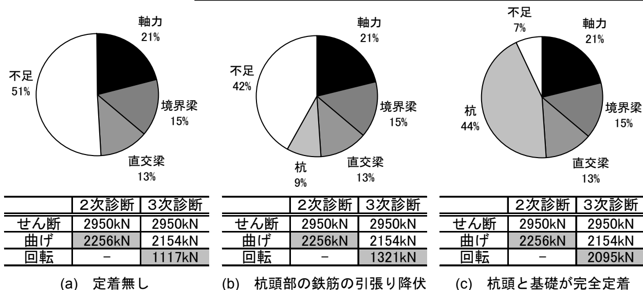
図－5 壁強度( \Sigma P_{wi} )に対する壁回転抵抗要因の寄与率 (略算法による結果。基礎重量は、軸力を含む。杭は基本形)
