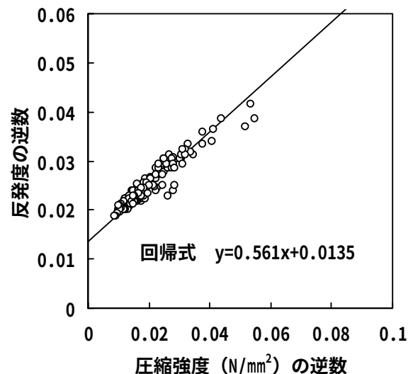
図-5 圧縮強度の逆数と反発度の逆数
