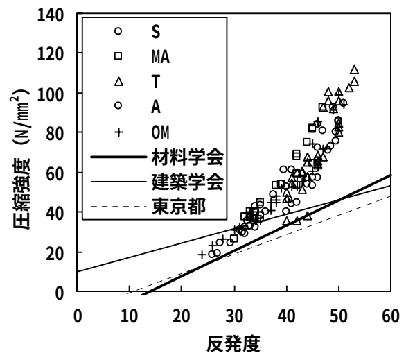
図-4 反発度と圧縮強度
