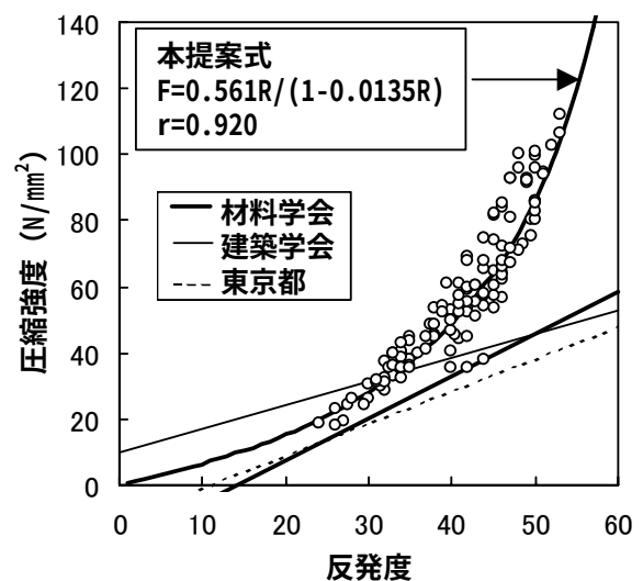
図-6 強度推定式
