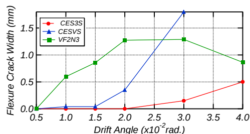
図－５ 最大残留曲げひび割れ幅
