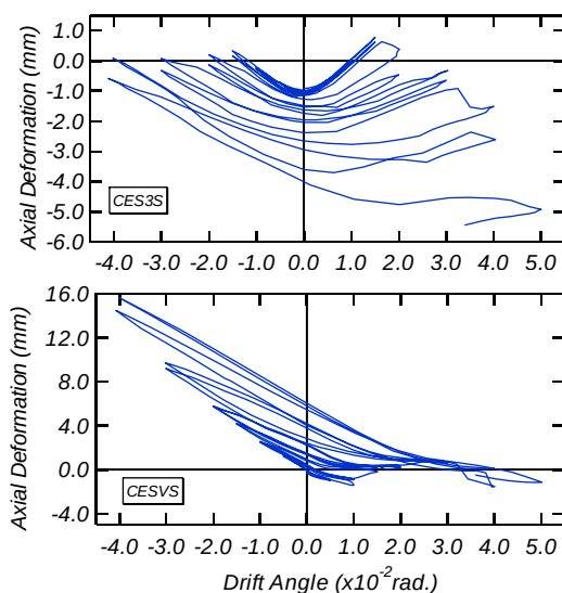
図－７ 軸方向変形
