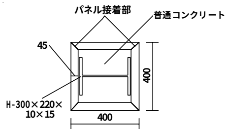
図-2 柱断面
