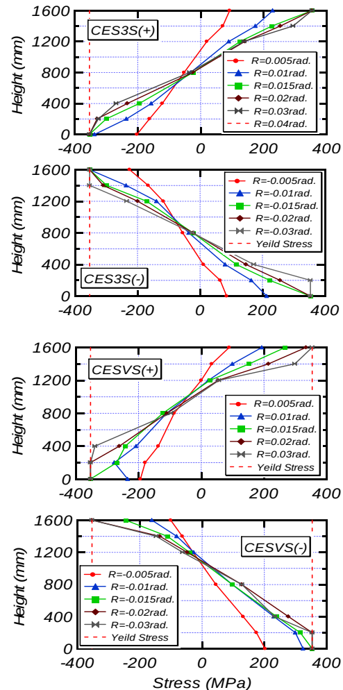
図-9 フランジ応力分布
