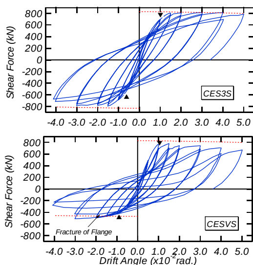
図－６ 荷重－変形関係
