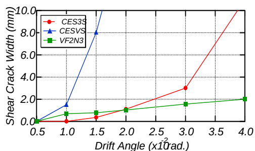
図－４ 最大残留せん断ひび割れ幅
