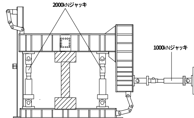
図－３ 載荷装置
