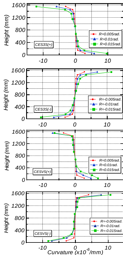
図－１０ 曲率推移
