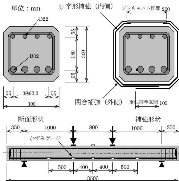
図－1 試験体形状と補強断面図
