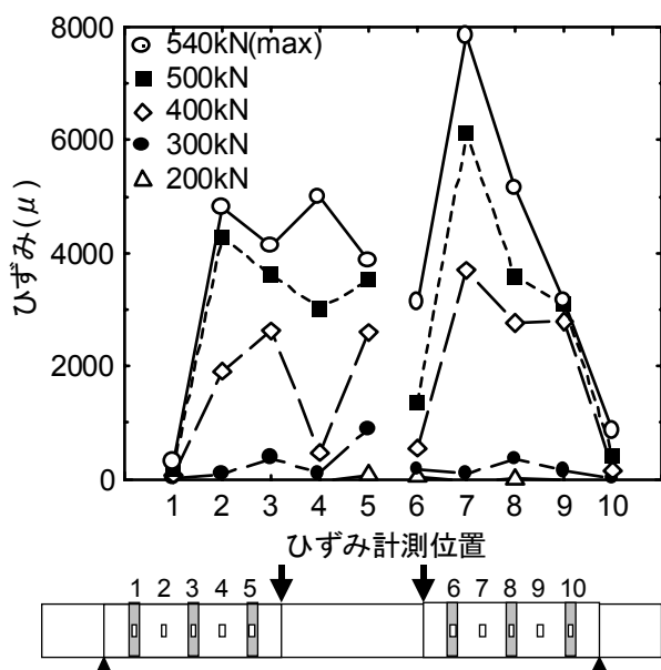
図－５ シートのひずみ分布 (AP2)
