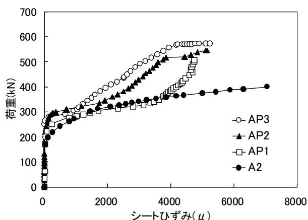
図－４ 荷重とシートひずみ関係
