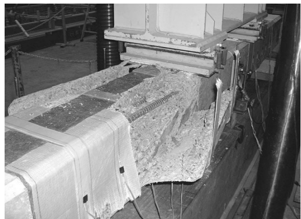
写真―2 破壊状況 (AP2)
