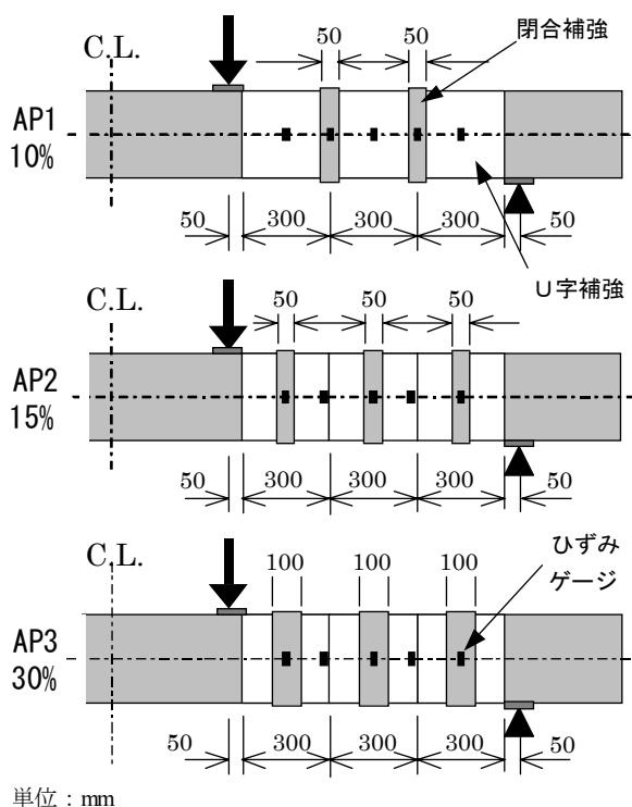
図－2 せん断補強概要
