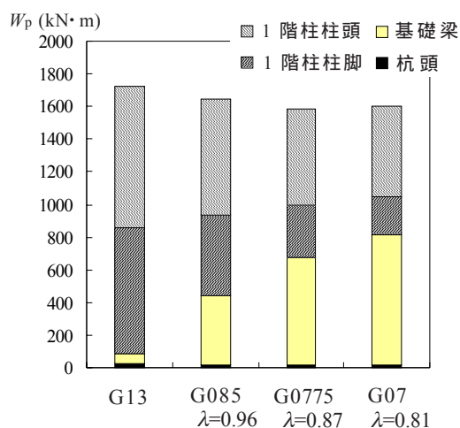
図 - 11 各部材の消費した履歴吸収エネルギー
