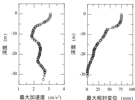
図-7 自由地盤の地震応答
