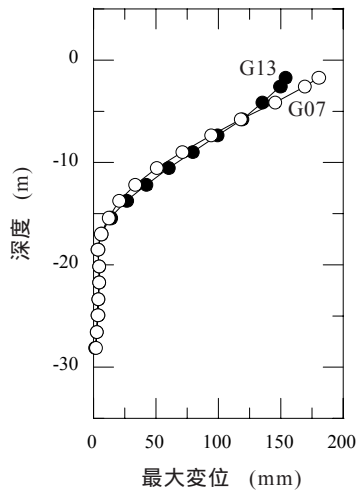
図 -13 地盤ばねの最大変位分布
