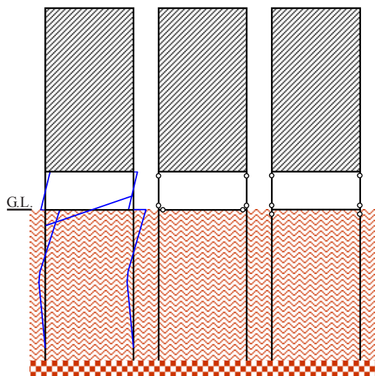
(1) モーメント図 (2) 基礎梁降伏 (3) 杭頭降伏 1)
