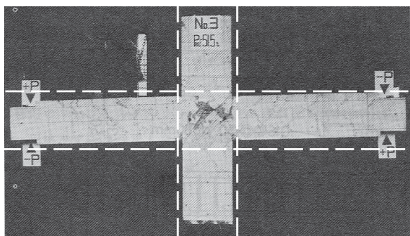
図-2 接合部破壊の例（JCI 選定試験体，マイクロデータその3） 4)
