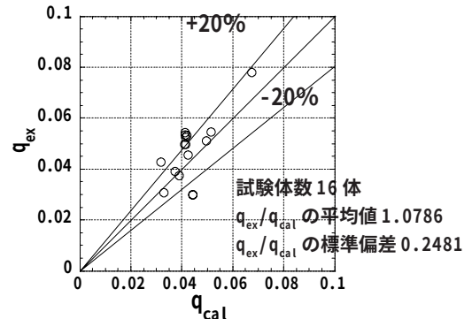
図-10 既往式による層せん断力解析値と実験値の比較
