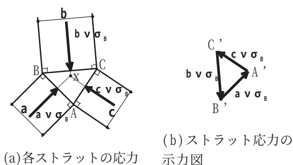
図-5 各ストラットの応力の関係図
