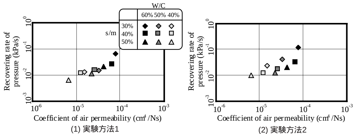
図-9 提案方法による結果と加圧法による結果との比較
