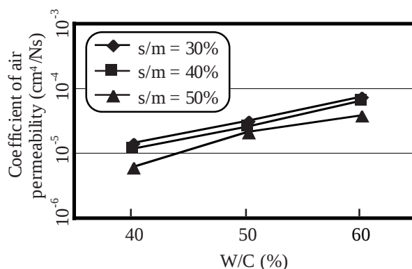
図-5 加圧法による透気係数
