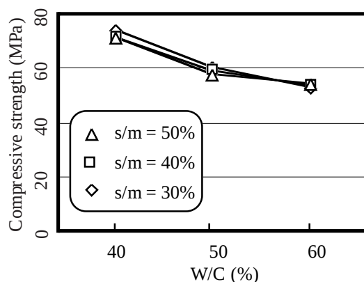
図-10 圧縮強度
