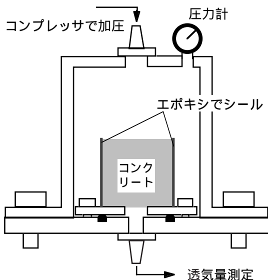
図-2 加圧法の概要
