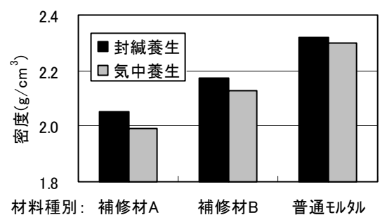
図-4 養生条件の違いによる密度
