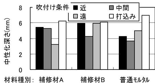
図-10 吹付け条件の違いによる中性化深さ
