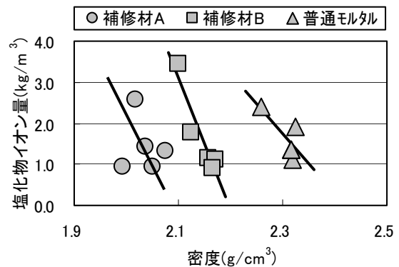
図-16 塩化物イオン量と密度の関係
