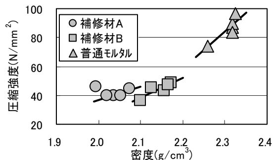
図-9 圧縮強度と密度の関係
