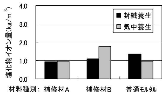
図-15 養生条件の違いによる塩化物イオン量
