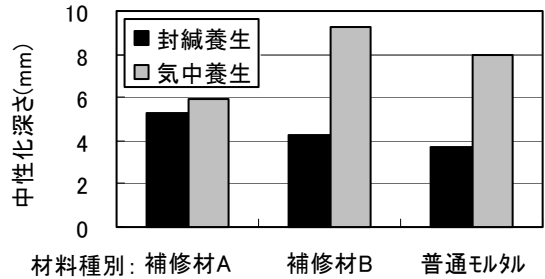
図-11 養生条件の違いによる中性化深さ
