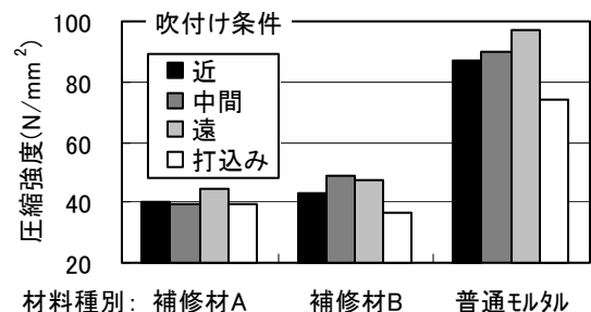
図-8 吹付け条件の違いによる圧縮強度
