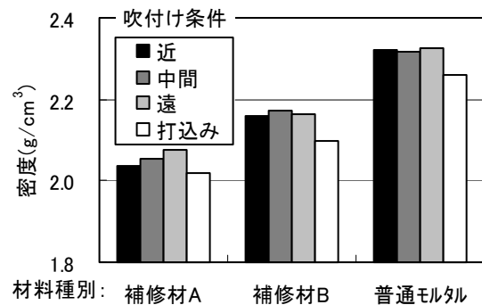
図-2 吹付け条件の違いによる密度
