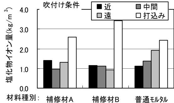
図-14 吹付け条件の違いによる塩化物イオン量
