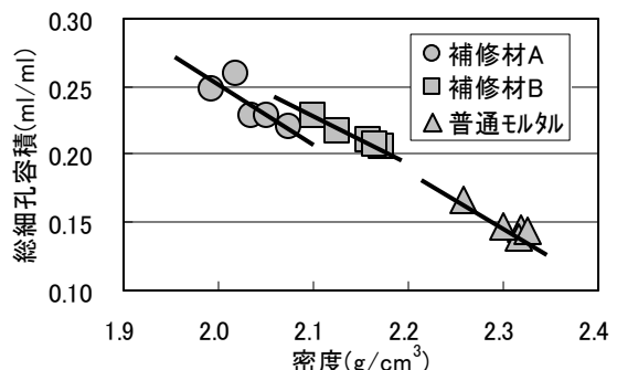
図-7 密度と総細孔容積の関係
