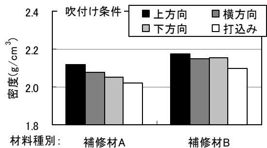
図-6 吹付け方向の違いによる密度
