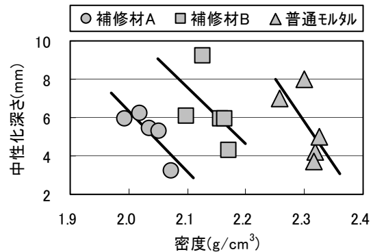
図-12 中性化深さと密度の関係
