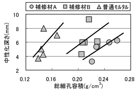
図-13 中性化深さと総細孔容積の関係
