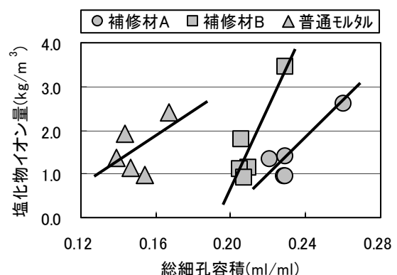
図-17 塩化物イオン量と総細孔容積の関係
