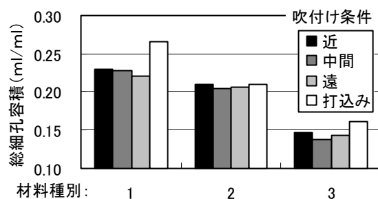
図-3 吹付け条件の違いによる総細孔容積
