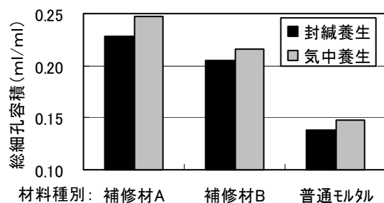
図-5 養生条件の違いによる総細孔容積
