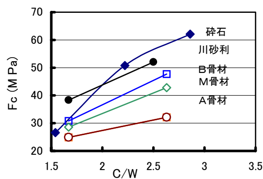
図-1 セメント水比と圧縮強度 (Fc)
