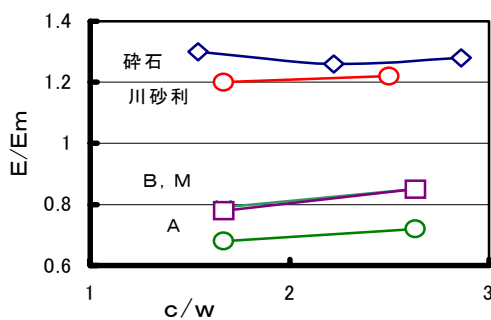
図 - 4 セメント水比と弾性係数比
