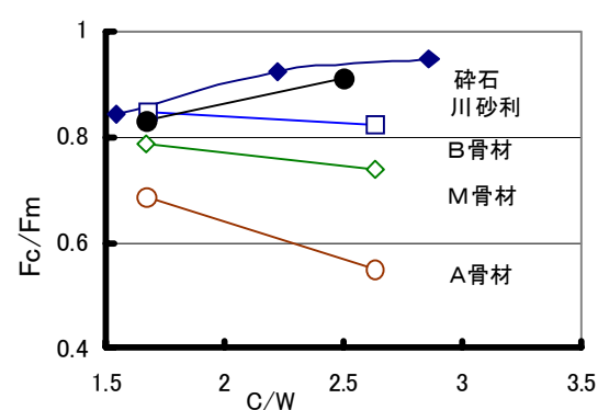
図-2 セメント水比 (C/W) と (Fc/Fm)
