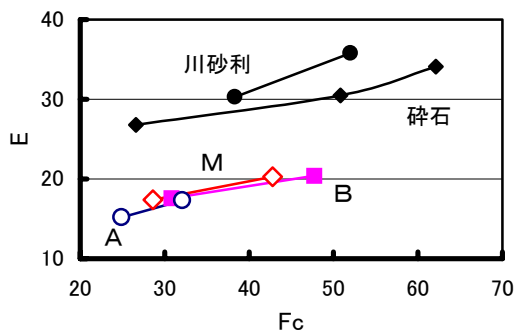
図 - 3 弾性係数と圧縮強度
