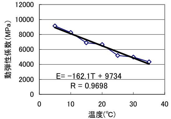
図－10 温度と動弾性係数の関係
