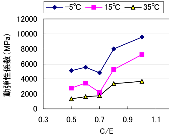
図－8 C／Eと動弾性係数の関係（複合体A）
