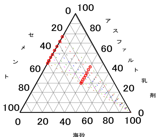
図-1 使用配合
