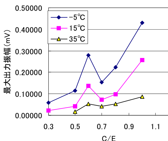
図-12 C/Eと最大出力振幅の関係 (複合体B)
