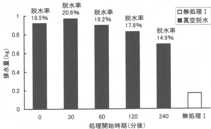
図-9 排水量(実験Ⅱ)
