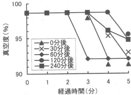
図-10 真空度の推移(実験Ⅱ)
