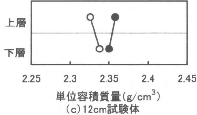
図-8 単位容積重量(実験Ⅰ)
