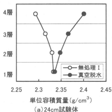
(a) 24cm試験体
