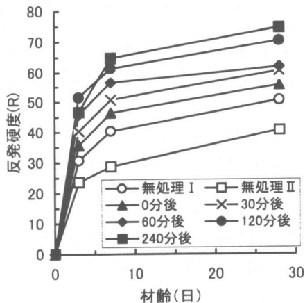
図-11 材齢と反発硬度の関係(実験Ⅱ)
