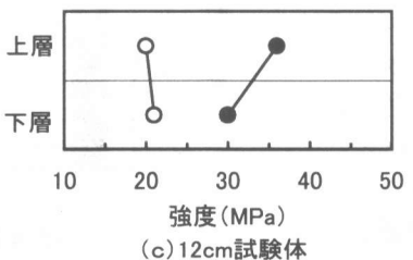
図-7 圧縮強度分布(実験Ⅰ)
