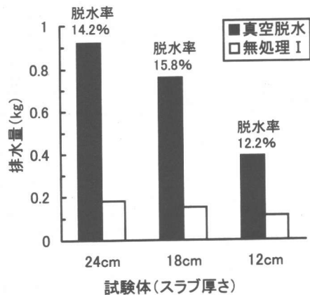
図-4 排水量(実験 I)
