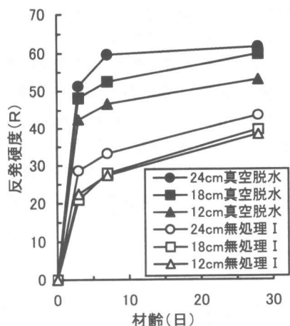
図-6 反発硬度と材齢の関係(実験Ⅰ)
