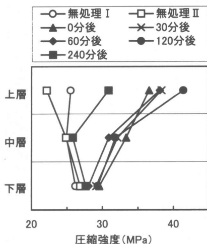
図-12 圧縮強度分布(実験 II)
