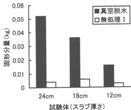
図-5 排水中の固形分量(実験 I)
