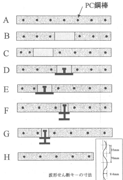
図-2 供試体の主な相違点
