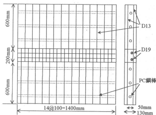
図-4 供試体Bの配筋図
