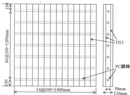
図-3 供試体Aの配筋図
