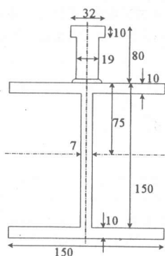
図-5 ジベル付きH型鋼の形状
