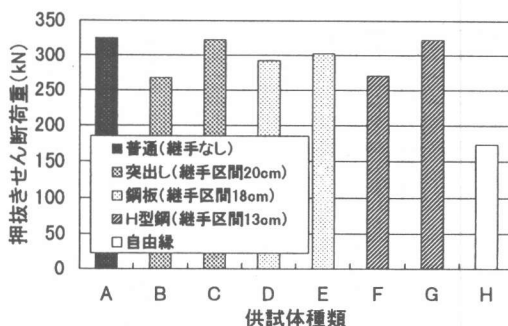
図-7 押抜きせん断強度試験結果
