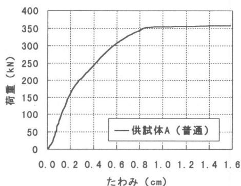
図-8 普通供試体の荷重—たわみ曲線
