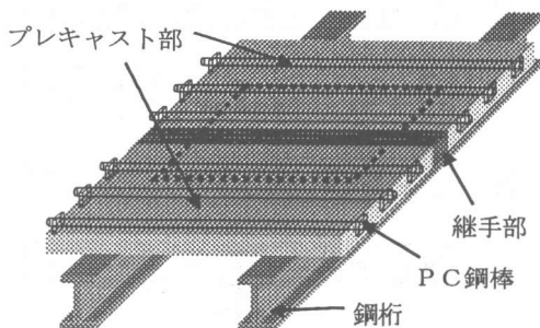
図-1 継手を有する床版例
