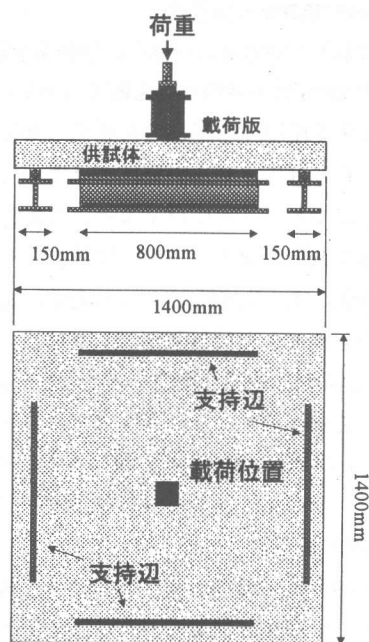
図-6 載荷方法
