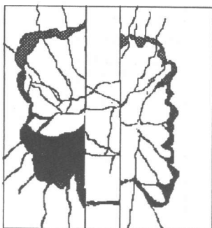
図-14 ひび割れ図 (せん断キー有り)
