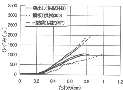
図-13 継手部主鉄筋の載荷板直下から20cm離れた位置のたわみとひずみの関係
