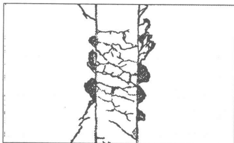
図-15 ひび割れ図 (せん断キー無し)
