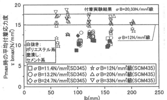
図6 \tau_{bmax} とlbとの関係
