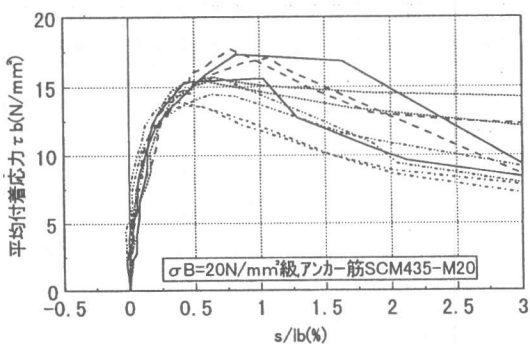
図8 lbを要因とした \tau_b -s/lb関係
