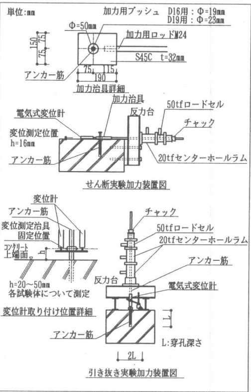
図2 加力装置図
