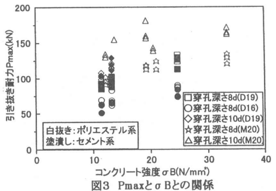
図3 Pmaxと \sigma_B との関係
