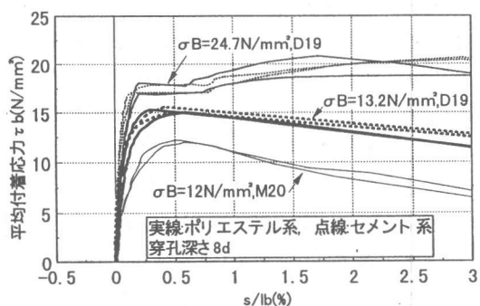
図9 \sigma_B を要因とする \tau_b -s/lb関係
