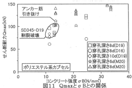
図11 QmaxとσBとの関係
