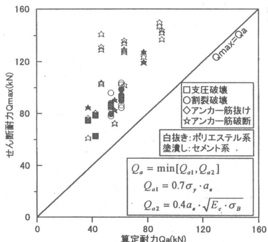
図13 実験結果と算定耐力との比較
