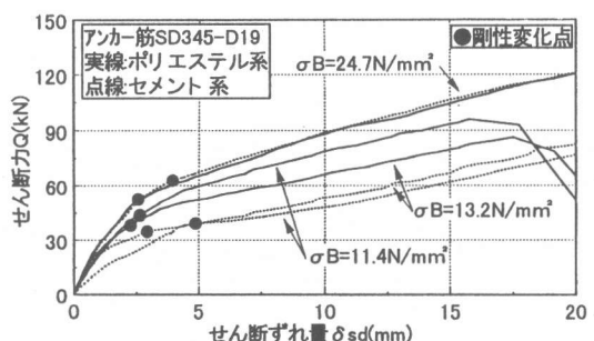
図14 σBを要因としたQ-δsd関係
