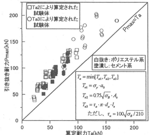
図5 実験結果と算定耐力との比較
