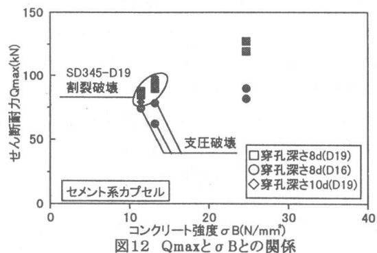
図12 QmaxとσBとの関係
