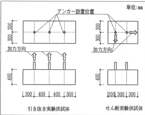
図1 コンクリートブロック供試体形状
