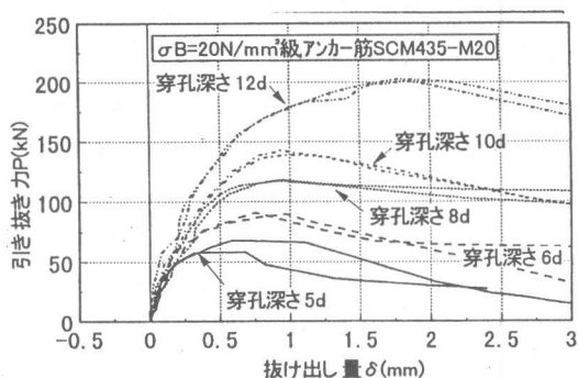
図7 引き抜き力-抜け出し量関係
