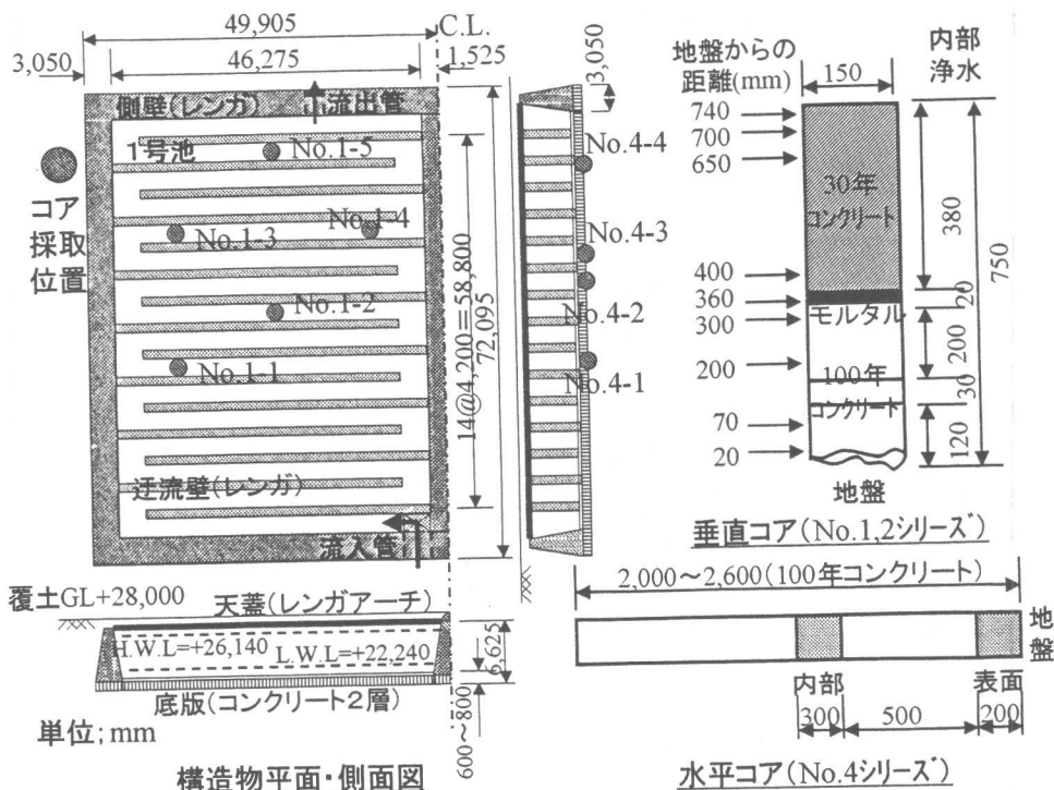
図-1 構造物の概要
