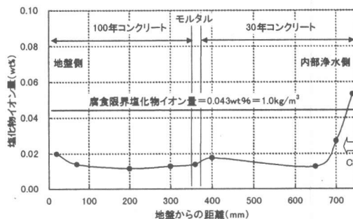
図-3 塩化物イオン量分布
