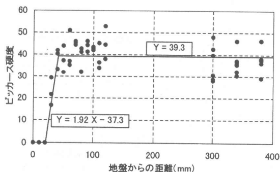
図-2 ビッカース硬度
