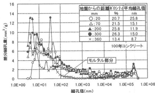
図-4 細孔径分布
