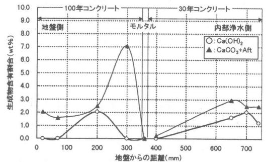
図-5 熱分析試験結果
