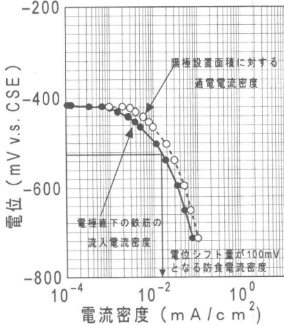
図-5 E-logI 試験結果 (Cl - =10kg/m 3 )
