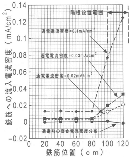
図-13 電流密度分布(10kg/m³)[鉛直]
