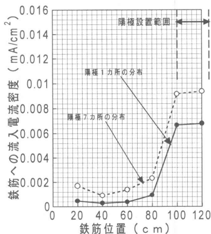
図-18 電流密度分布と陽極設置数の関係( Cl^- = 5\text{kg/m}^3 )
