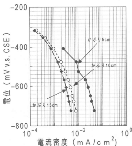
図-7 電流密度とかぶりの関係 ( Cl^{-}=5\text{kg/m}^3 )
