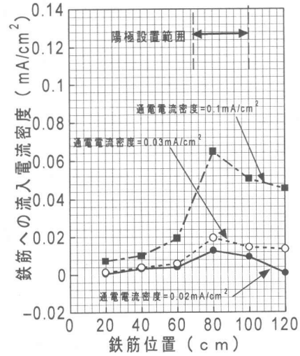
図-14 電流密度分布(10kg/m³)[水平]
