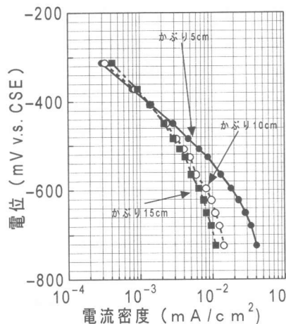
図-6 電流密度とかぶりの関係 ( Cl^{-}=1\text{kg/m}^3 )
