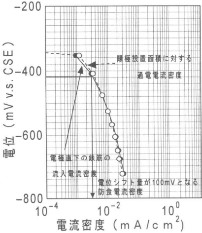
図-4 E-logI 試験結果 (Cl - =5kg/m 3 )
