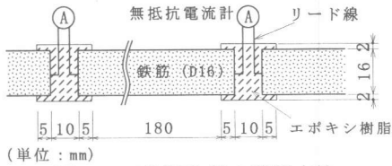
図-2 分割鉄筋の接続方法
