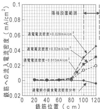
図-11 電流密度分布( 5\text{kg/m}^3 )[鉛直]
