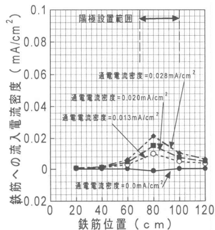
図-12 電流密度分布( 5\text{kg/m}^3 )[水平]
