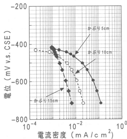
図-8 電流密度とかぶりの関係 ( Cl^{-}=10\text{kg/m}^3 )
