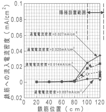
図-9 電流密度分布( 1\text{kg/m}^3 )[鉛直]
