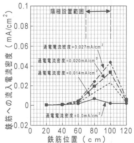
図-10 電流密度分布( 1\text{kg/m}^3 )[水平]
