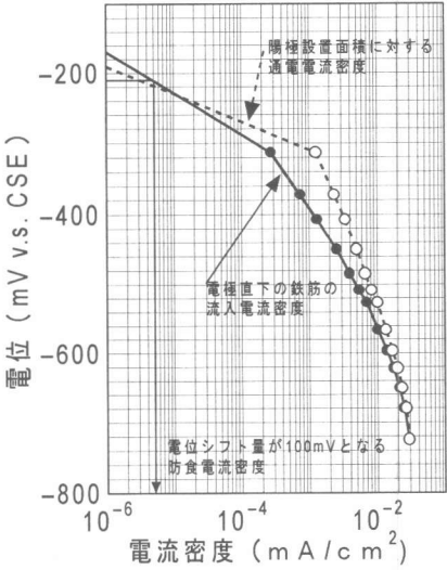
図-3 E-logI 試験結果 (Cl - =1kg/m 3 )
