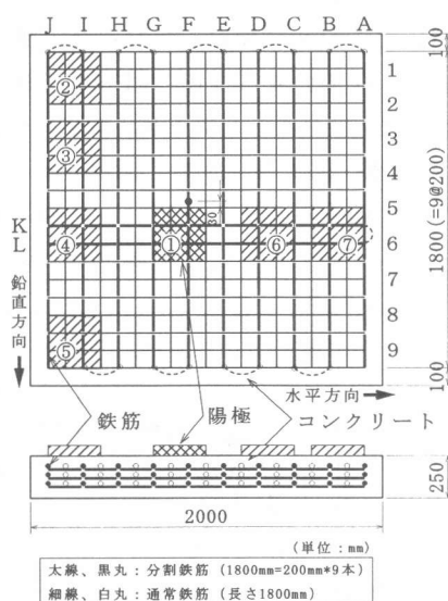
図-1 供試体の形状と鉄筋の配置
