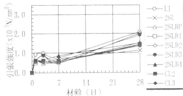
図-9 引張強度試験結果
