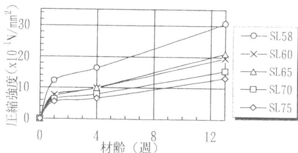
図-2 水/消石灰比
