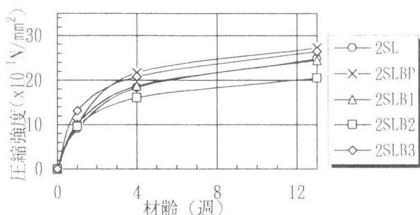
図-4 消石灰：細骨材+レンガ比 1:2.00
