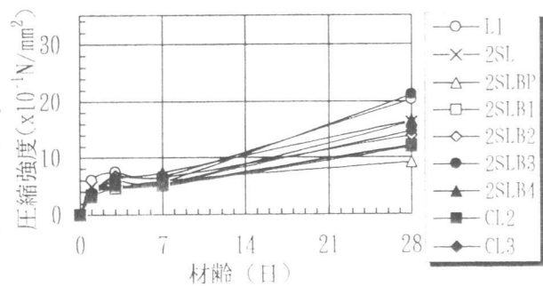
図-8 圧縮強度試験結果
