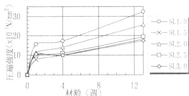
図－1 消石灰：細骨材比
