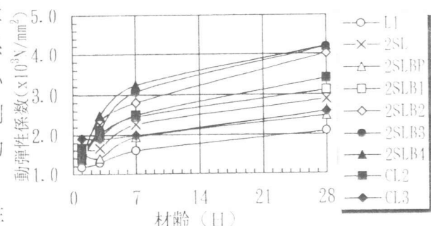
図-10 動弾性係数試験結果
