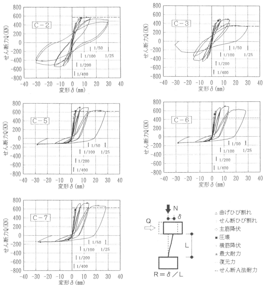
図-5 荷重-変形関係
