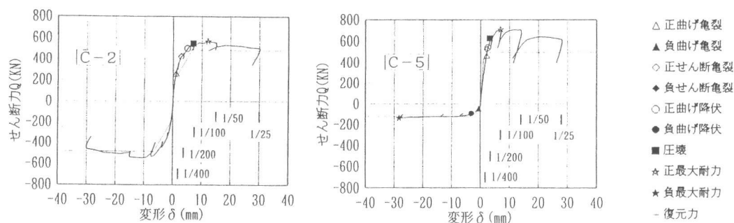
図-7 復元力特性解析結果例
