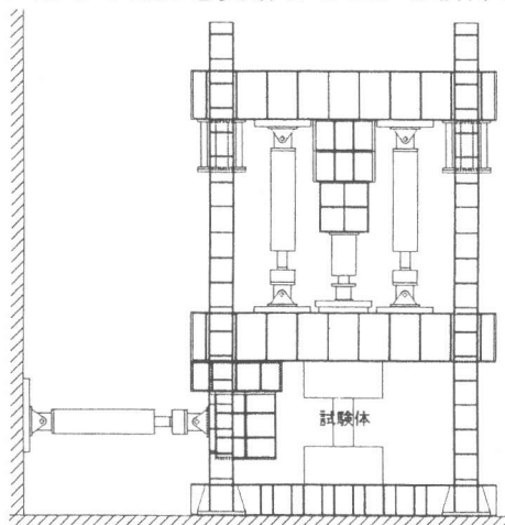
図-2 加力装置
