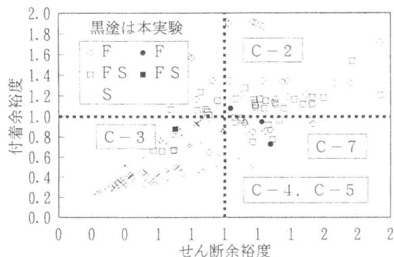
図-6 余裕度と破壊モードの関係
