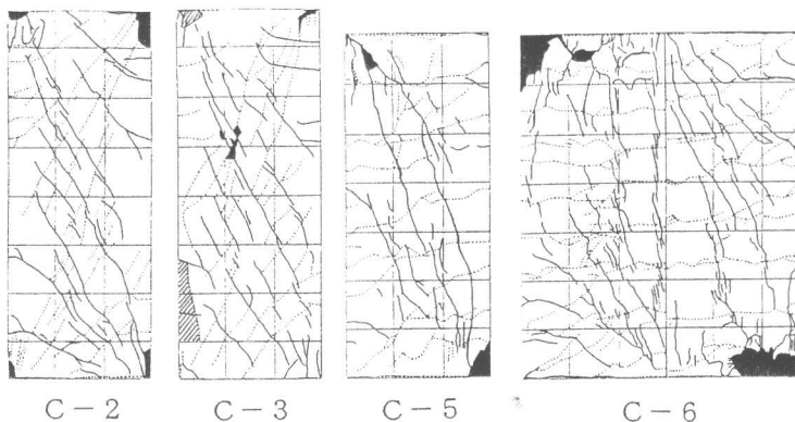
図-4 1/50rad時ひび割れ性状
