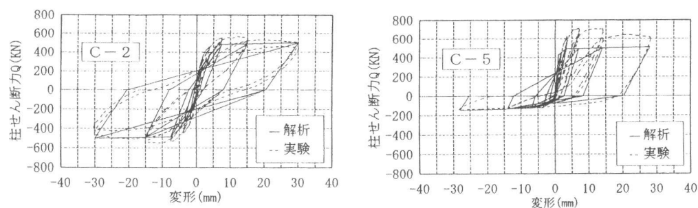
図-8 繰返し解析結果例
