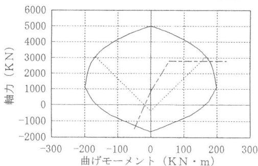
図-3 M-N载荷曲線
