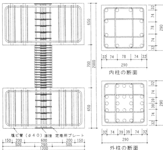
図-1 試験体形状及び配筋例
