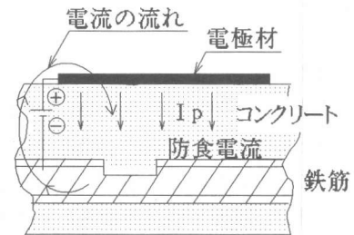
図-3 防食電流の流れ
