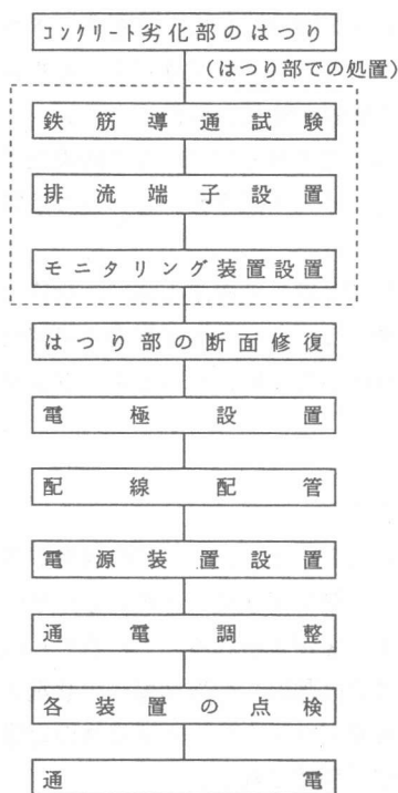
図-7 施工手順
