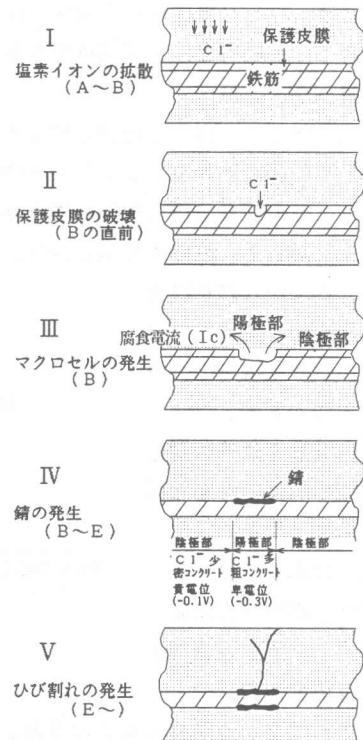
図-1 鉄筋の腐食プロセス
