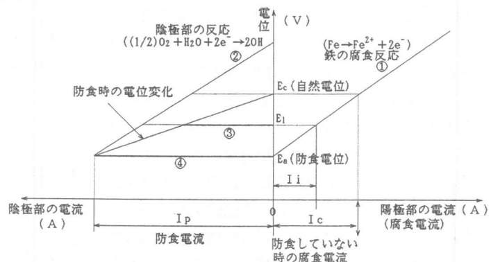
図-4 鉄筋腐食と電気防食の原理
