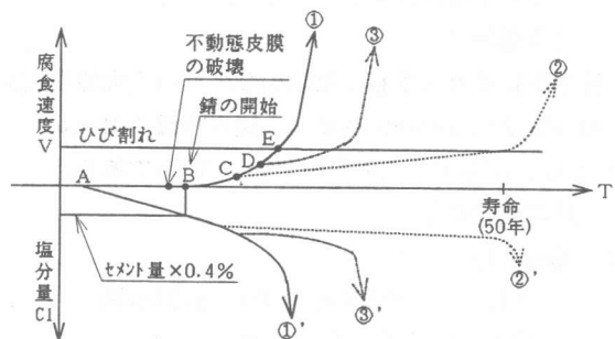
図-2 腐食速度、塩分量と経年変化
