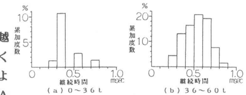
図-19 非腐食模型第17段階目のAE継続時間分布状態(荷重増加時)
