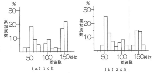
図-22 AE周波数分布状態
