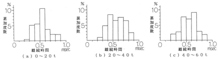
図-17 非腐食模型中央1点載荷時のAE継続時間分布状態(荷重増加時)
