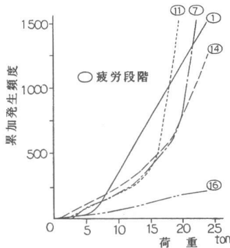
図-7 AE累加発生頻度 （非腐食，荷重時）
