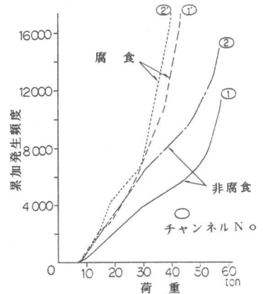
図-6 AE累加発生頻度（荷重時）
