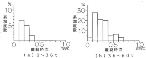
図-20 腐食模型第17段階目のAE継続時間分布状態(荷重増加時、再載荷時含まず)
