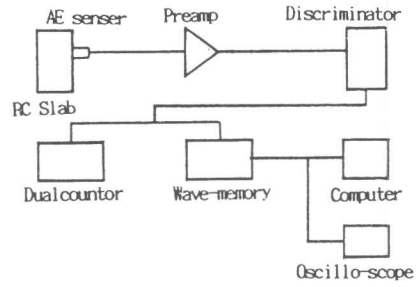
図-3 計測システム
