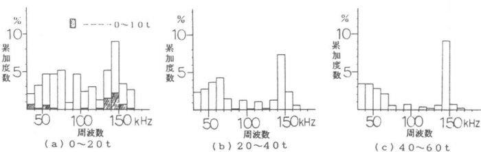
図-12 非腐食模型中央1点載荷時のAE周波数分布状態（荷重増加時）
