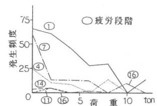
図-10 AE発生頻度 （腐食，除荷時）
