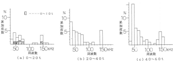
図-13 腐食模型中央1点載荷時のAE周波数分布状態（荷重増加時、再載荷時含まず）
