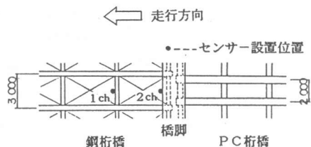
図-21 センサー設置位置
