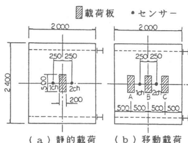
図-2 荷重板, センサー位置 (単位, mm)
