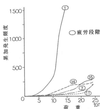
図-8 AE累加発生頻度 （腐食，荷重時）
