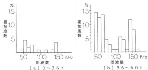
図-14 非腐食模型第17段階目のAE周波数分布状態（荷重増加時）
