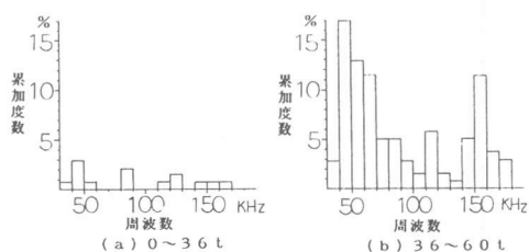
図-15 腐食模型第17段階目のAE周波数分布状態（荷重増加時、再載荷時含まず）
