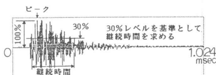
図-16 AE継続時間の整理方法
