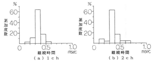
図-23 AE継続時間分布状態
