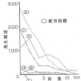
図-9 AE発生頻度 （非腐食，除荷時）
