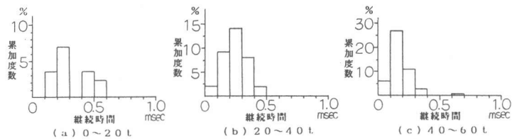
図-18 腐食模型中央1点載荷時のAE継続時間分布状態(荷重増加時、再載荷時含まず)
