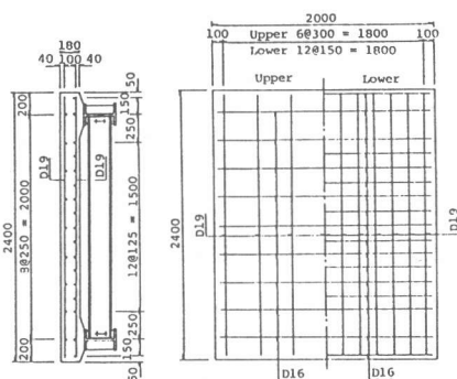
図-1 RC床版模型 (単位, mm)
