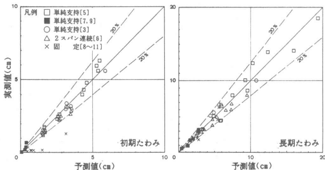
図3 たわみ実測値と予測値の対応
