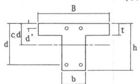
図2 T形断面の I_g 計算に必要な諸元
