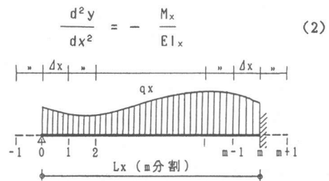
図1 はり材の分割と節点番号
