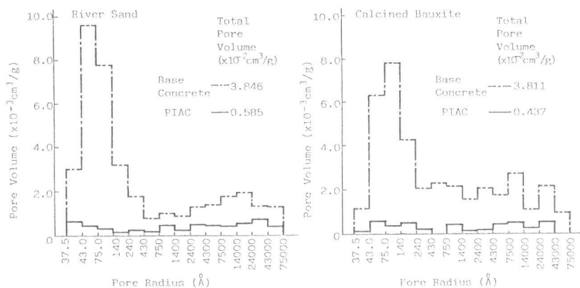
図-3 250℃で乾燥した基材コンクリート及びポリマー含浸オートクレーブ養生コンクリートの細孔径分布
