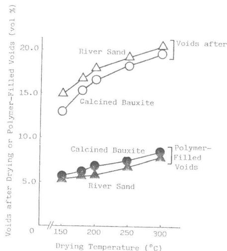
図-1 乾燥温度と基材コンクリートの乾燥後の空けき率とポリマー充てん率の関係
