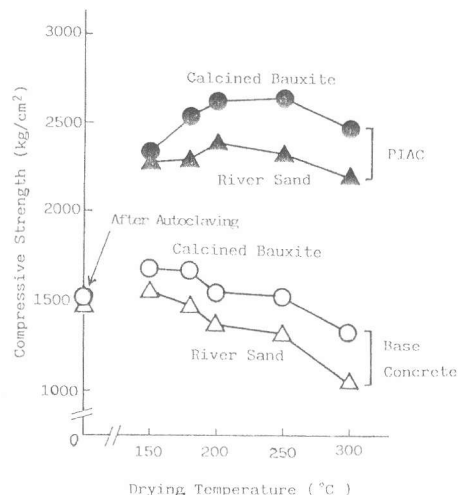
図-2 乾燥温度と基材コンクリート及びポリマー含浸オートクレーブ養生コンクリートの圧縮強度の関係
