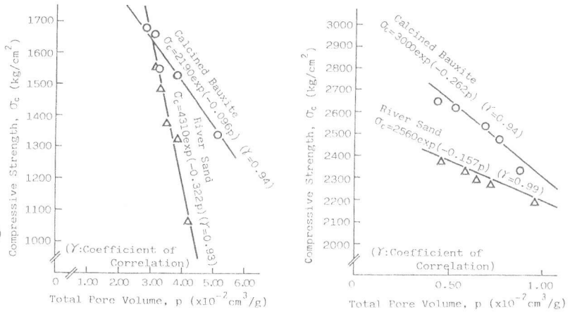
図-4 基材コンクリート及びポリマー含浸オートクレーブ 養生コンクリートの圧縮強度と全細孔容積の関係
